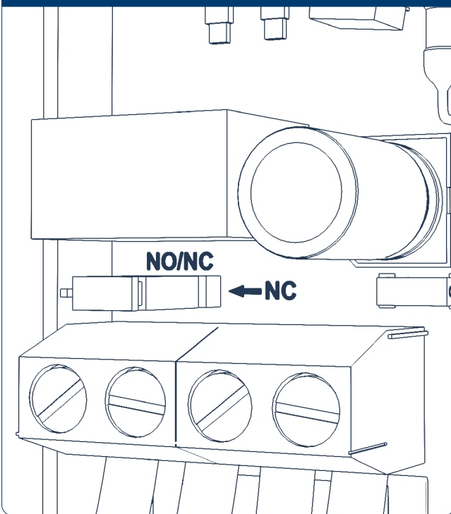
Рис. 39. Фотозащитный элемент. Положение переключателя — NC
