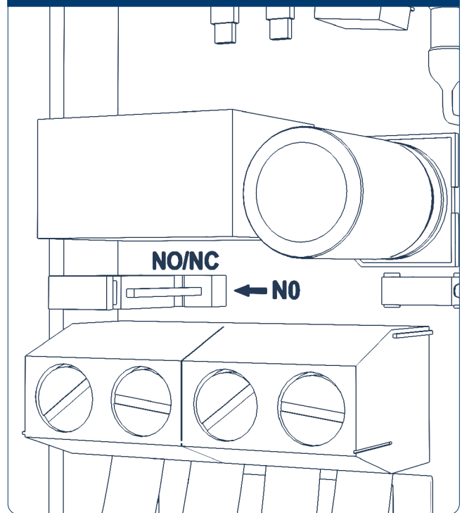
Рис. 40. Фотозащитный элемент. Положение переключателя — NO
